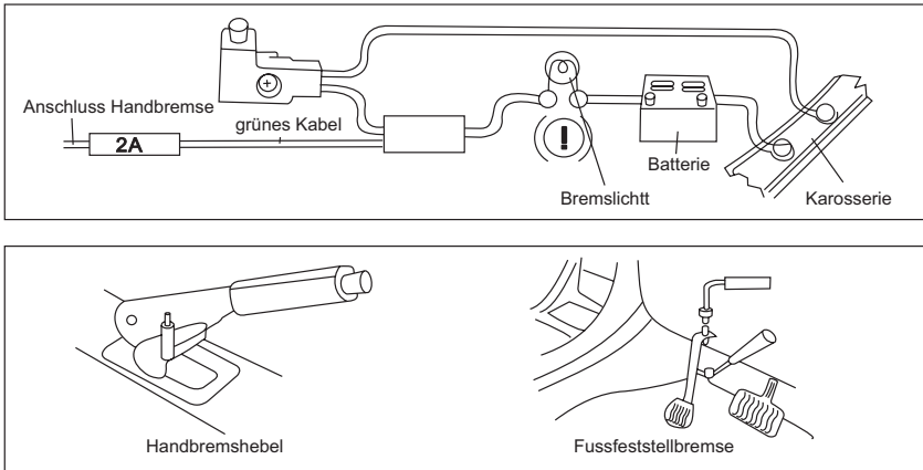
Abbildung 2: Handbremssystem: Kabelanschlüsse
