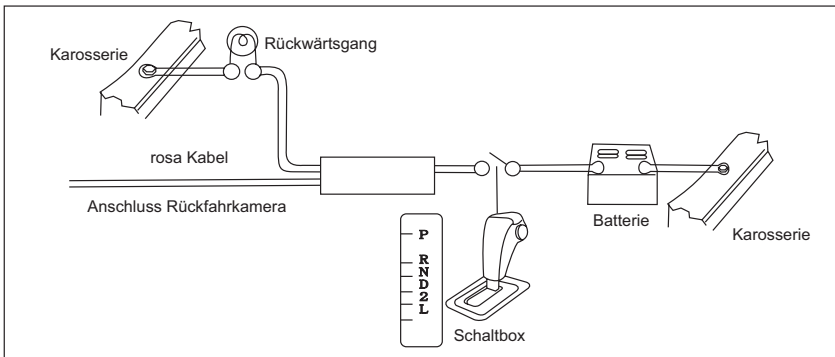
Abbildung 3: Rückwärtsgang: Kabelanschlüsse
